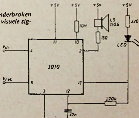
Fig. 2. Signalering met regelbaar referentie niveau.
